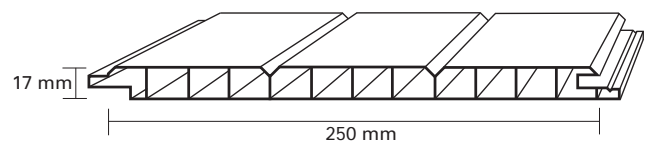
PVC-Hohlkammerprofil D250-17
