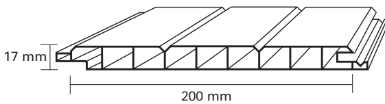
PVC Hohlkammerprofil D200-17
