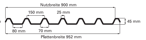
Profil 45/150 - PVC
