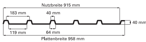
Profil 40/183 - PVC
