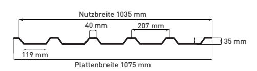
Profil 35/207 - PC
