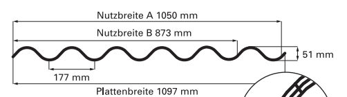
Profil 177/51 - P6,5 - Hohlkammer - PC
