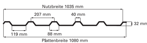
Profil 35/207 Fischer alt - PVC
