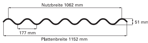
Profil 177/51 - P6,75 - PVC
