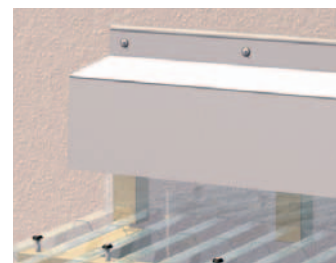
C Kappliste (Z-Profil) (bauseits)
