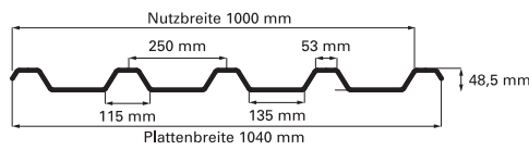
Profil 50/250 - PVC
