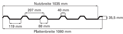
Profil 35/207 Fischer neu - PVC
