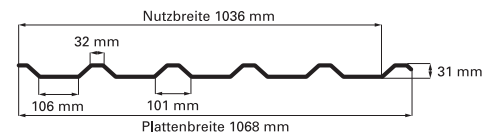
Profil 35/207 Arcelor - PVC
