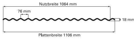
Profil 76/18 - PVC
